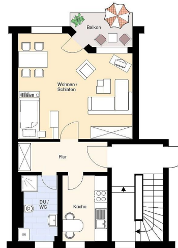
Grundriss möbliert
